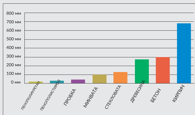
Толщины различных материалов при одинаковой теплоизоляции
