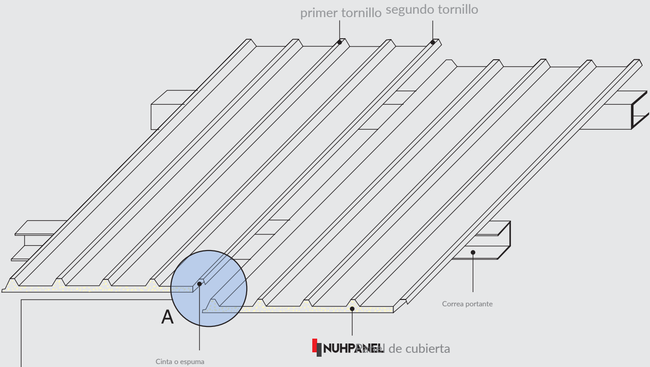
DETALLE EN EL PUNTO A
