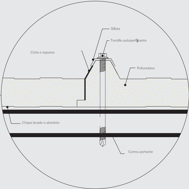
DETALLE EN EL PUNTO A
