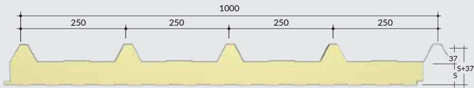
PANEL DE CUBIERTA ACÚSTICO HÍBRIDO
