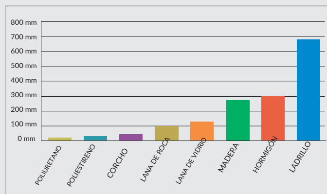
Es espesores de distintos materiales con el mismo aislamiento térmico
