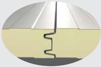
DETALLE DE UNIÓN
